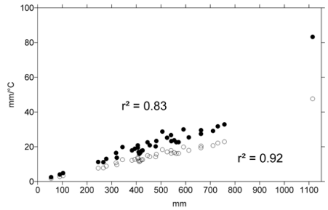
Figura 6. Regresión entre la lluvia media anual de Sonora (eje X) y sus correspondientes valores de los índices de aridez de Lang (puntos) y De Martonne (círculos) (eje Y). Los coeficientes de determinación para cada par de series (siendo mayor el coeficiente entre el índice De Martonne y la lluvia) se indican en la figura.
