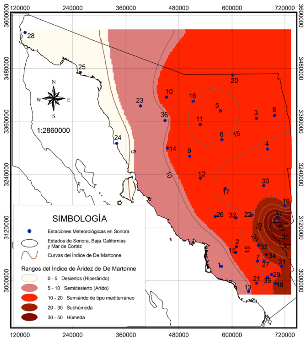
Figura 5. Igual que la figura 4, pero para el Índice de De Martonne
