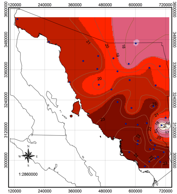
Figura 2. Isotermas medias anuales para el estado de Sonora calculadas en el periodo 1920-2011.
