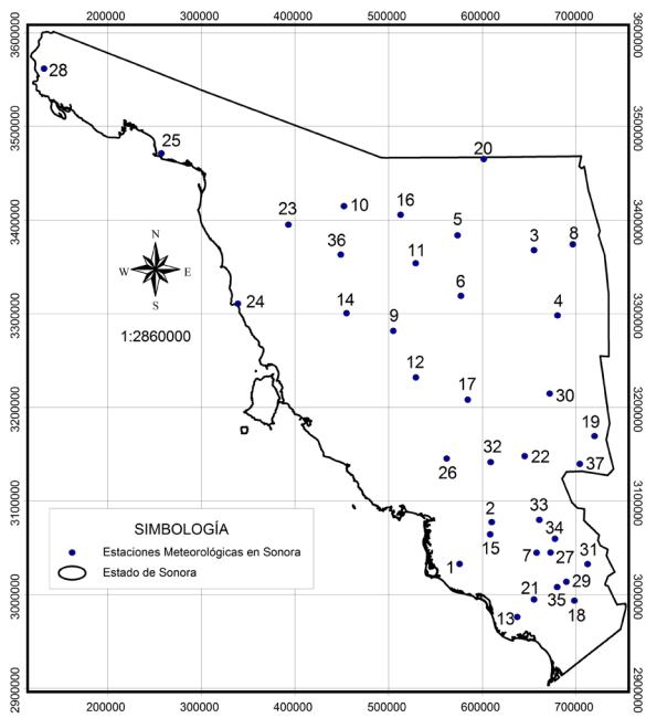
Figura 1. Ubicación de las Estaciones Meteorológicas seleccionadas en el Estado de Sonora.
