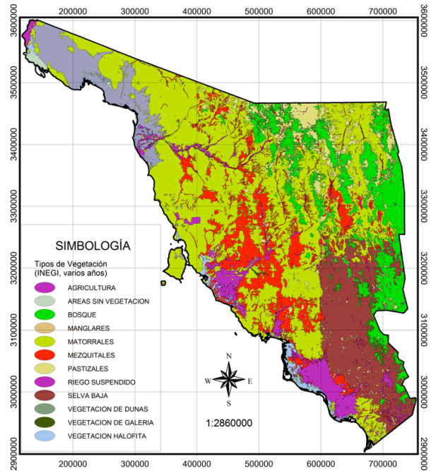
Figura 7. Vegetación del estado de Sonora según información de INEGI (2006).
