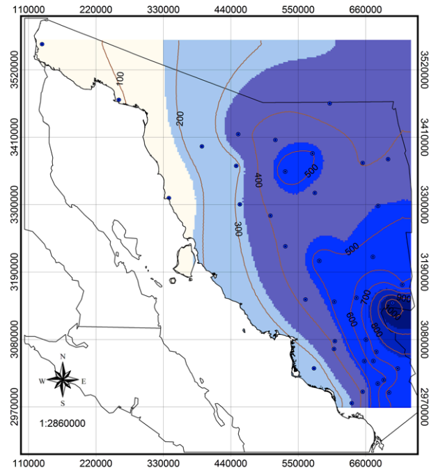
Figura3. Isoyetas medias anuales calculadas en el periodo 1920-2011
