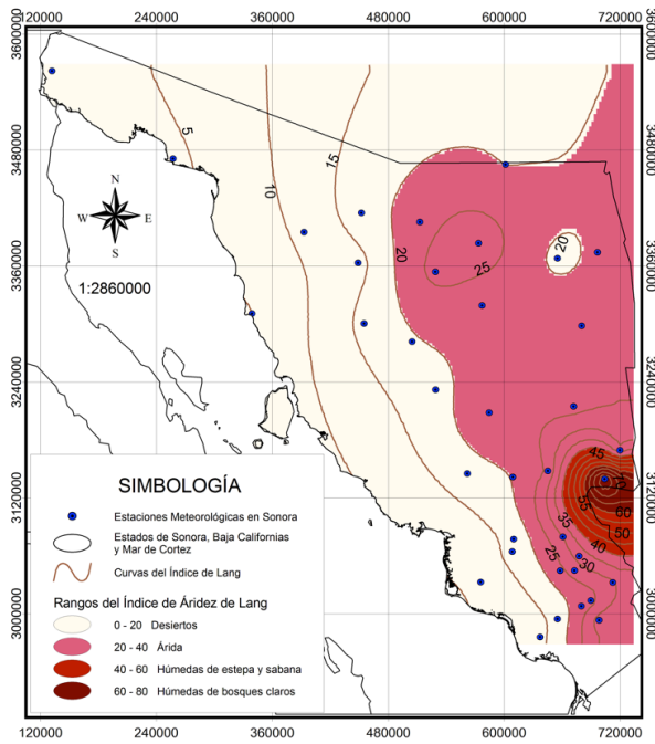
Figura 4. Distribución de los valores del Índice de Lang calculados para el estado de Sonora con datos entre 1920 y 2011.
