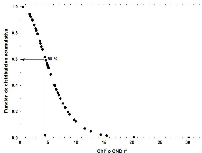
FIGURA 2. Función de distribución acumulada de \chi^2 con seis grados de libertad para obtener el valor crítico teórico de DNC r^2 en el arreglo S^5 asociado al 60 % de la población (subpoblación de bajo rendimiento).
