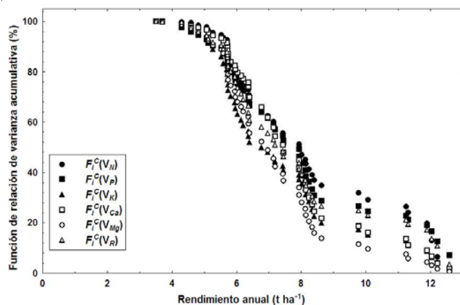
FIGURA 1. Relaciones cúbicas experimentales entre el rendimiento en Chile, cultivar Caribe o Chiltepín de C. frutescens , y las funciones de proporción de varianza acumulada en el arreglo S 5 para estimar el punto de inflexión y el rendimiento crítico para separar a las sub-poblaciones de alto y bajo rendimiento.
