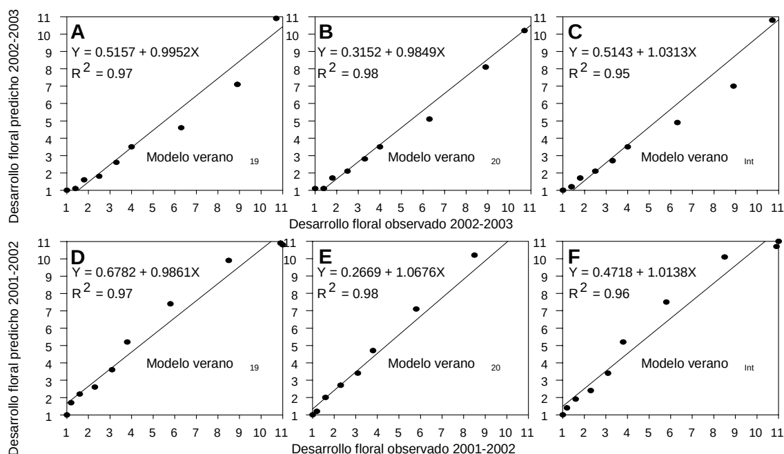
FIGURA 2. Ajuste de valores entre el estado de desarrollo floral de aguacate 'Hass' observado (evaluación directa) y el estado de desarrollo floral predicho empleando los modelos verano 19 (A), verano 20 (B) y verano Int. (C), obtenidos durante 2001 a 2002 para brotes del flujo de verano, para predecir el estado de desarrollo floral en el año 2002 a 2003, así como los los modelos verano 19 (D), verano 20 (E) y verano Int. (F) obtenidos en el 2002 a 2003 para predecir el estado de desarrollo floral en el año 2001 a 2002. Escala de desarrollo floral (Salazar-García et al. , 1998): 1 = yema cerrada y puntiaguda; 11 = antesis.
