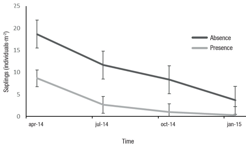
Figure 4. Density of saplings in presence and absence of livestock over the years in a queñoa ( Polylepis australis ) forest at Parque Provincial Potrero de Yala (Jujuy, Argentina). Figura 4. Densidad de renovales en presencia y ausencia del ganado a lo largo del tiempo en un bosque de queñoa ( Polylepis australis ) en el Parque Provincial Potrero de Yala (Jujuy, Argentina).
