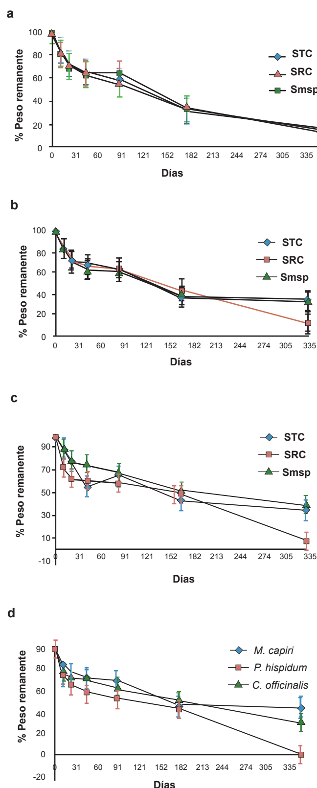
FIGURA 2. Peso restante de a) Robinsonella mirandae , b) Robinsonella mirandae/Coffea arabica , c) Mezcla de hojarasca y d) Mastichodendron capirii , Piper hispidum y Croton officinalis , en el Sistema Tradicional de Café (STC), Sistema Rústico de Café (SRC) y Selva mediana subperennifolia (Smsp) de San Miguel, Veracruz, México.
